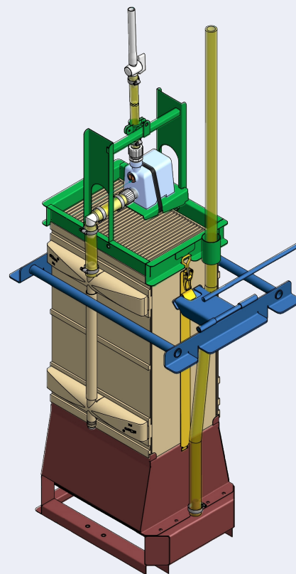
GEP membraanfilter
